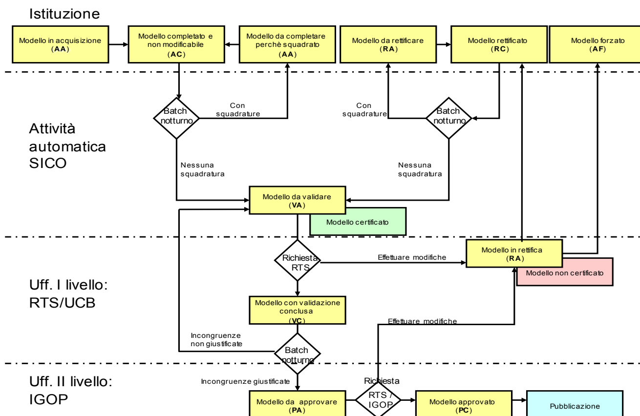
Figura 7 - Processo dei dati in SICO
